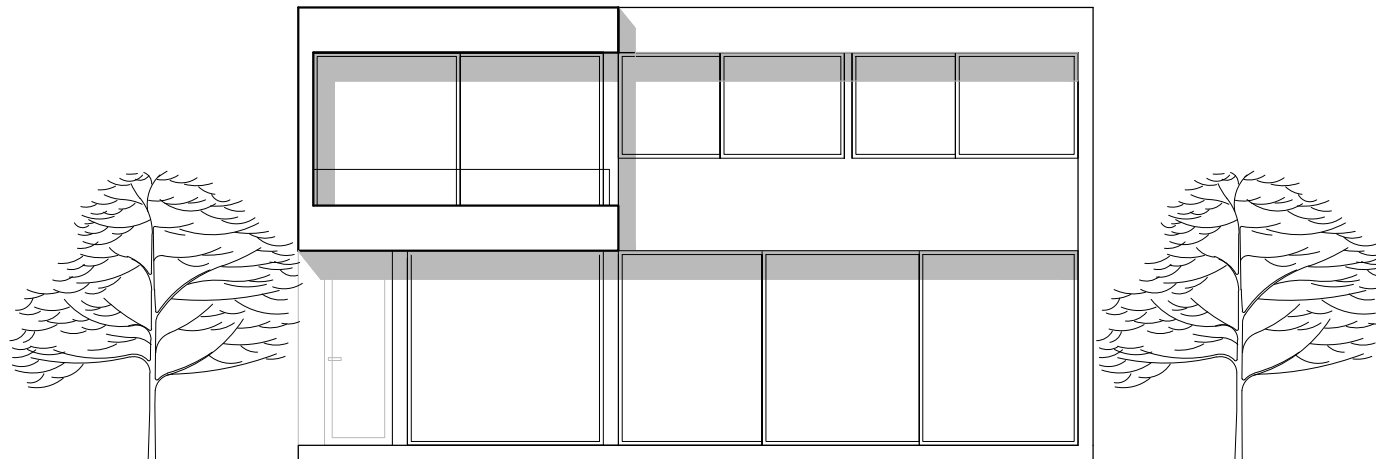
ELEVACION JARDIN
